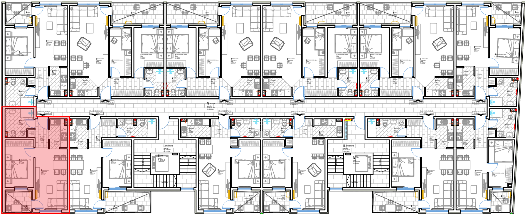
POLOŽAJ STANA 33 U OBJEKTU NA SPRATU 3
