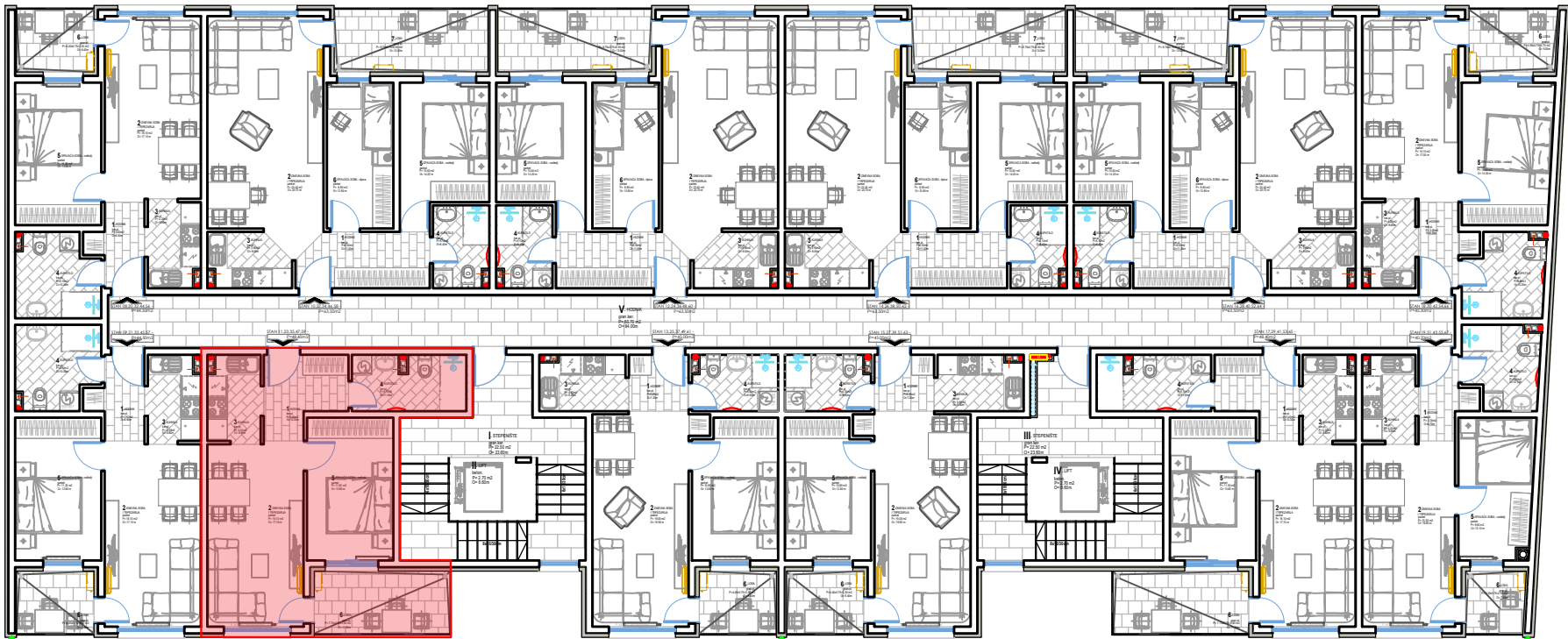
POLOŽAJ STANA 59 U OBJEKTU NA SPRATU 5
