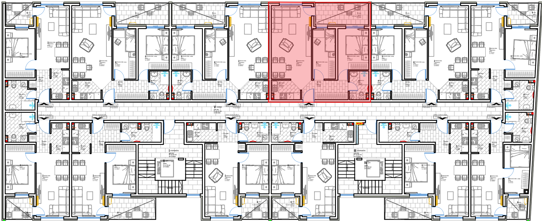
POLOŽAJ STANA 26 U OBJEKTU NA SPRATU 2
